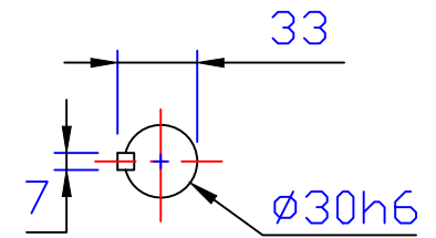
出力轴 Output Shaft
