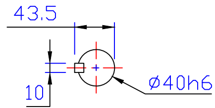
出力轴 Output Shaft
