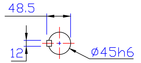
出力轴 Output Shaft
