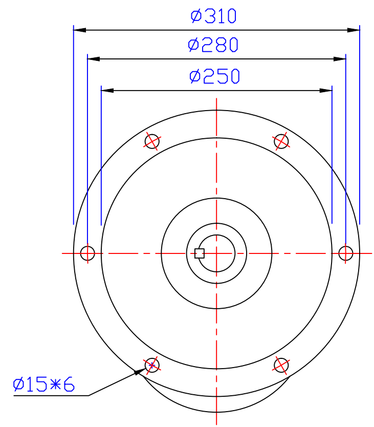
出力轴 Output Shaft
