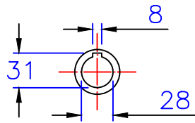
入力孔 Input hole
