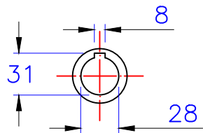
入力孔 Input hole
