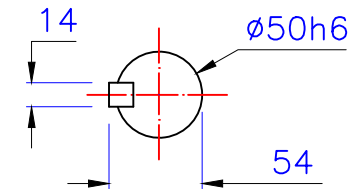
出力轴 Output shaft
