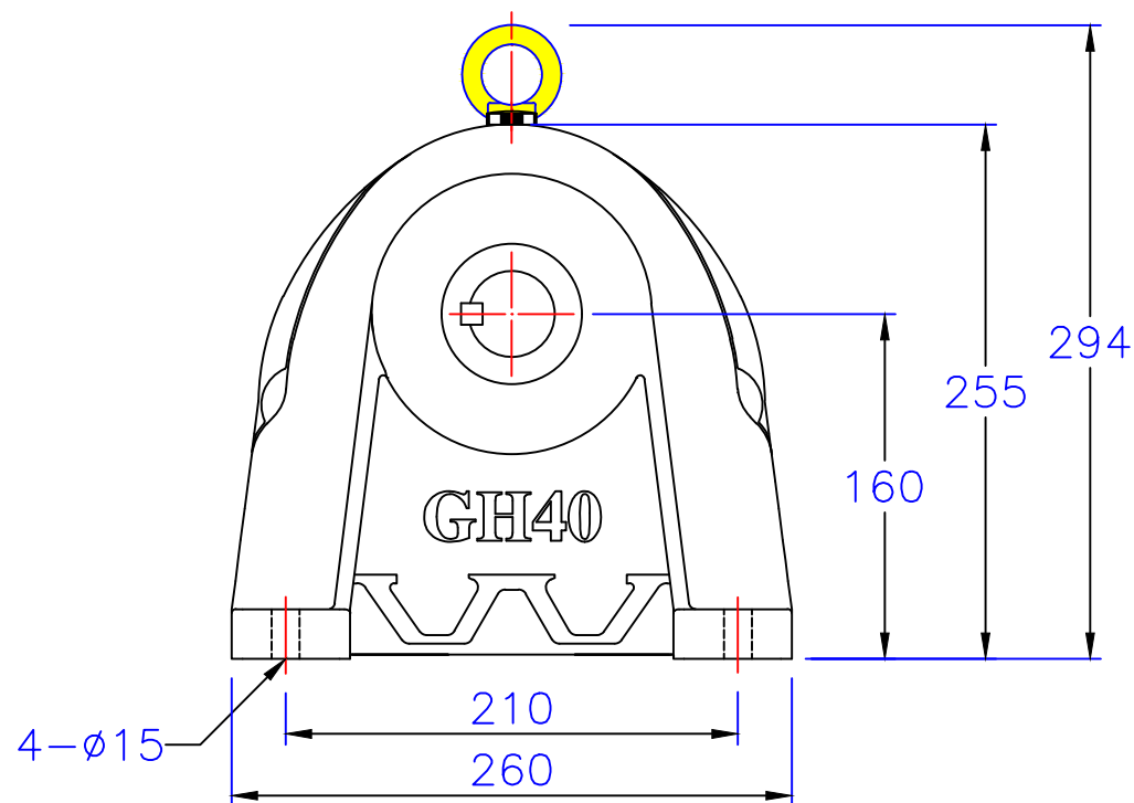
出力轴 Output shaft
