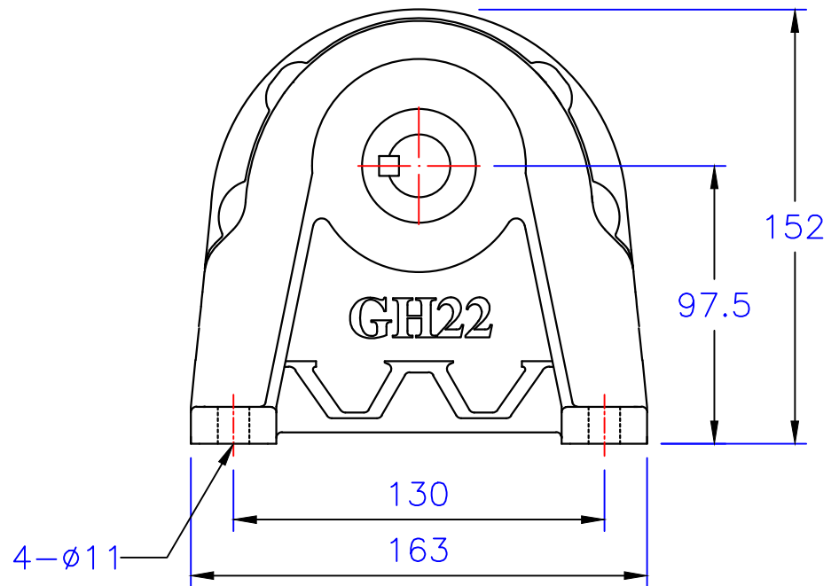
出力轴 Output shaft
