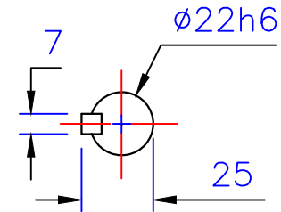
出力轴 Output shaft
